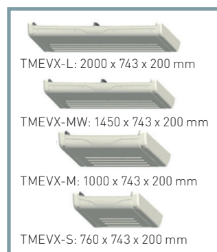
Verdampfer
